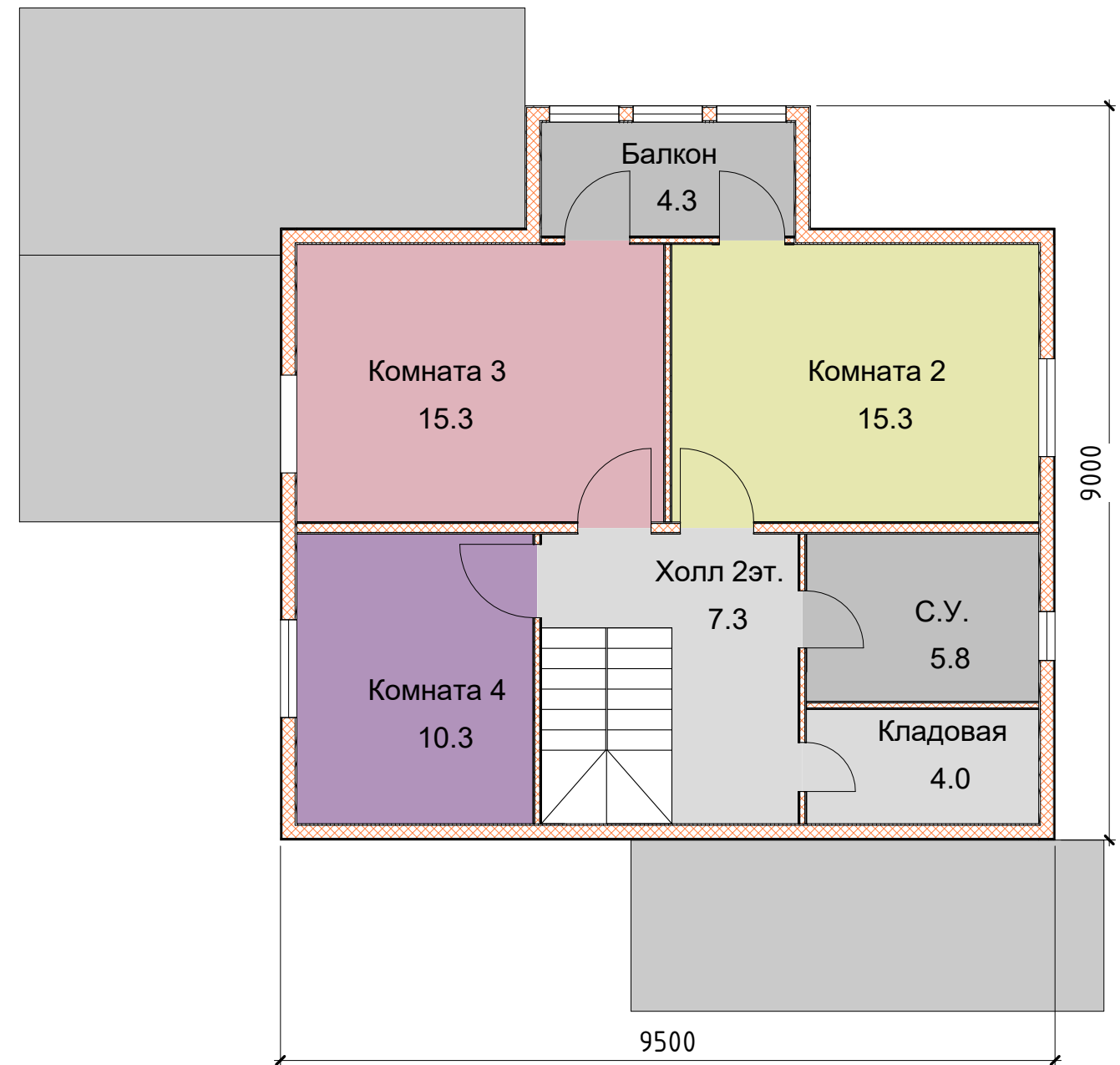
2 Этаж
