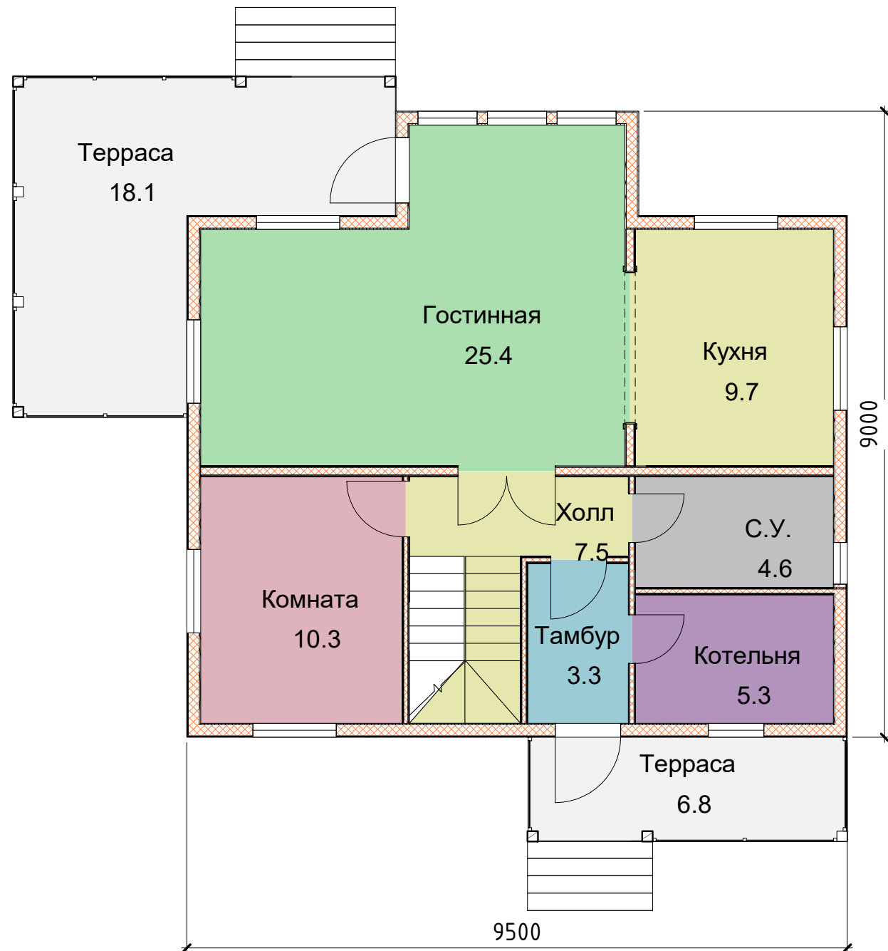
1 Этаж
